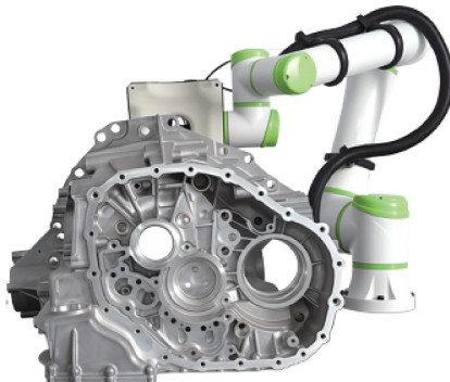
配合机械臂多角度, 多方位检测缺陷及瑕疵
