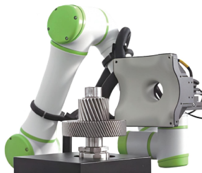
配合机械臂, 飞拍检测旋转齿轮缺陷
